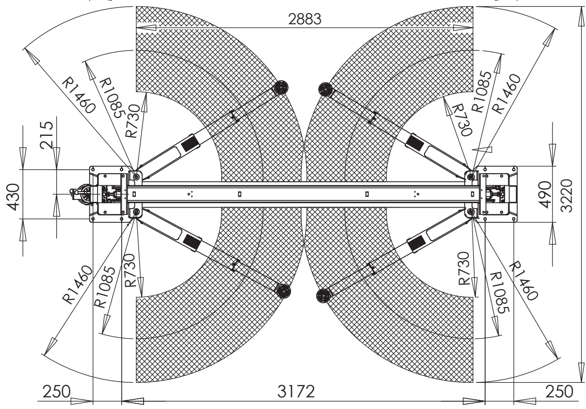
BN-6250WP 加高单边解锁外接龙门
