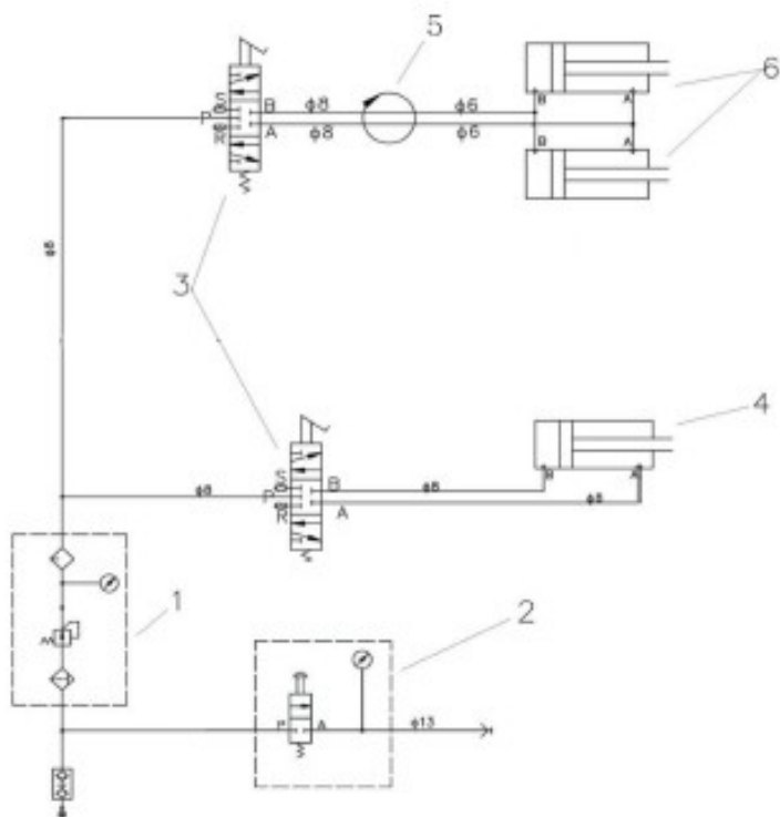
Схема пневмосистемы
