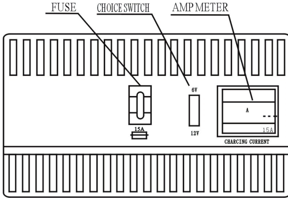
Frontplattenzeichnung
