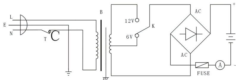
Электрическая схема
