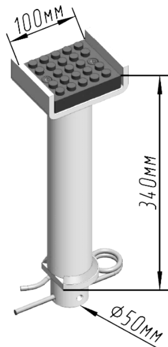
Рисунок 1 - Адаптер в сборе
